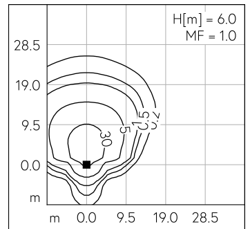
LED 4000 K 117 W 14320 lm-h H = 6 m / CIE Flux 39 80 99 100 100 / A30 selon DIN ...
