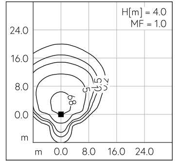
LED 4000 K 117 W 14320 lm-h H = 4 m / CIE Flux 39 80 99 100 100 / A30 selon DIN ...
