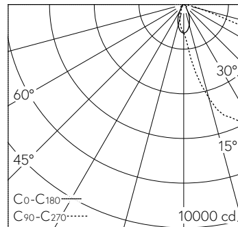
LED 4000 K 117 W 14320 lm-h H = 6 m / CIE Flux 39 80 99 100 100 / A30 selon DIN ...
