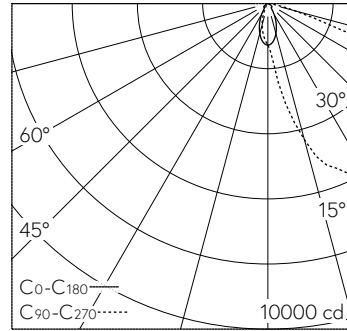
LED 4000 K 117 W 14320 lm-h H = 4 m / CIE Flux 39 80 99 100 100 / A30 selon DIN ...
