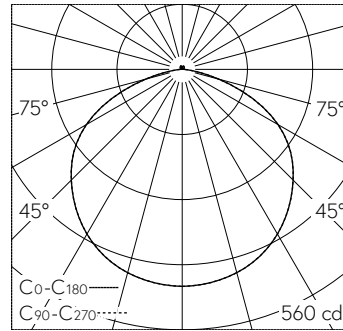
LED 4000 K 16 W 1439 lm-h / CIE Flux 46 79 97 98 100 / A42 selon DIN 5040
