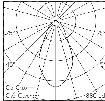
LED 3000 K 9.2 W 857 lm-h / CIE Flux 71 90 97 93 100 / A62 selon DIN 5040
