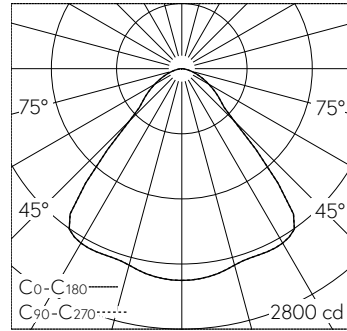
LED 3000 K 41 W 4576 lm-h 86° / CIE Flux 71 92 99 100 100 / A60 selon DIN 5040
