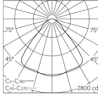
LED 4000 K 41 W 4340 lm-h 86° / CIE Flux 71 92 99 100 100 / A60 selon DIN 5040
