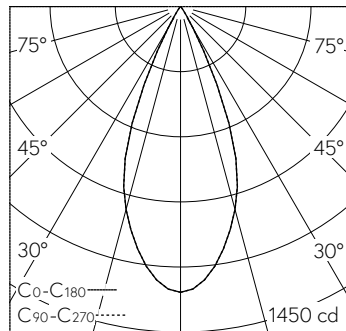
LED 4000 K 7.5 W 571 lm-h 42° / CIE Flux 99 100 100 100 100 / A80 selon DIN 5040
