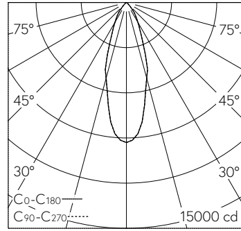
LED 34.2 W 3532 lm-h 126° Indirekt / CIE Flux 44 76 96 100 100 / A40 selon DIN 5040
