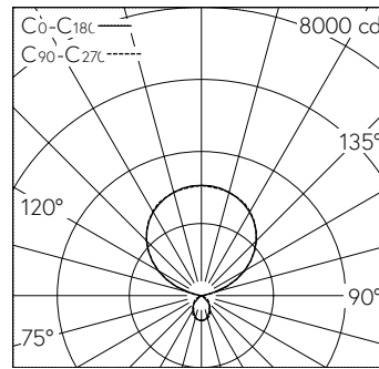
LED 2700 – 6500 K 83 W 9870 lm-h / CIE Flux 66 92 98 12 100 / D63 selon DIN 5040
