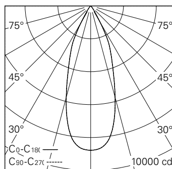
LED 4000 K 31 W 3913 lm-h 38° / CIE Flux 98 100 100 100 100 / A80 selon DIN 5040
