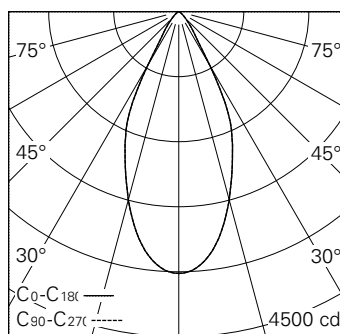
LED 3000 K 27 W 2228 lm-h 48° / CIE Flux 94 99 100 100 100 / A80 selon DIN 5040
